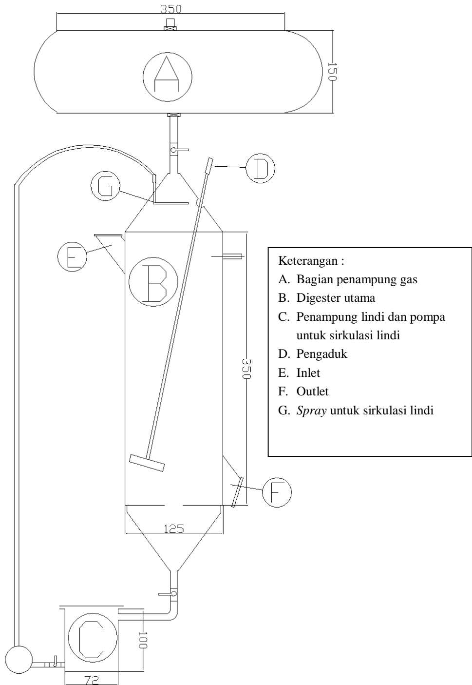
Gambar 17. Rancangan Biogas
