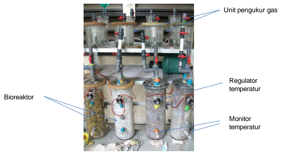
Gambar 5. Foto reaktor biogas 10 L
