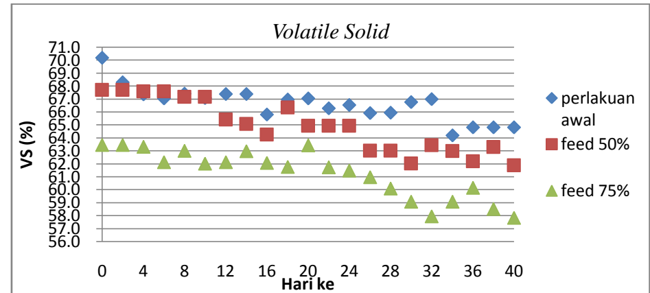
Gambar 14. Perubahan Bahan Organik ( Volatile Solid )
