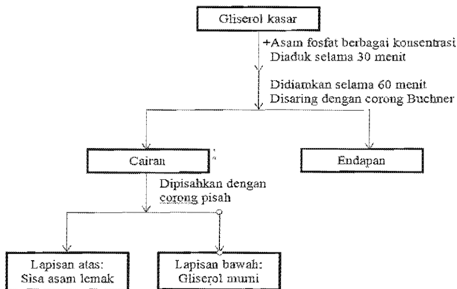
Gambar 1 Diagram alir proses pemurnian gliserol
