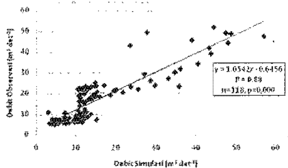
Gambar 5. Debit harian simulasi setelah validasi dan dan debit harian observasi (bulan Februari-Maret tahun 2009 dan 2011)
