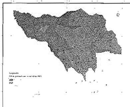
Gambar 8. Aliran permukaan (mm) tahun 2011
