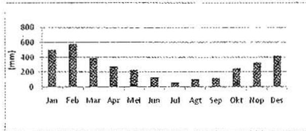
Gambar 1. Rata-rata curah hujan tahun 2008-2011
