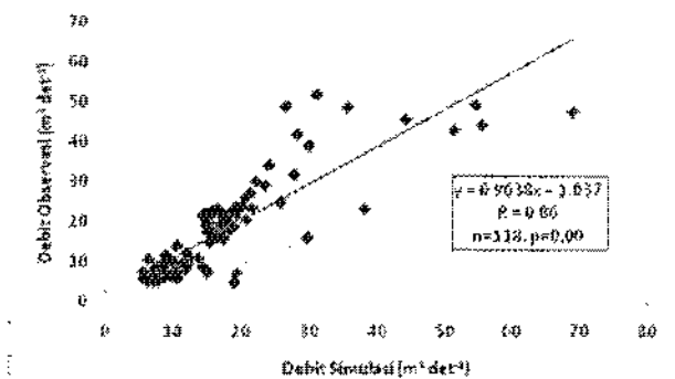
Gambar 3. Debit harian simulasi sebelum validasi dan dan debit harian observasi (bulan Februari-Maret tahun 2009 dan 2011)
