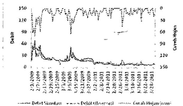
Gambar 2. Hidrograph aliran simulasi sebelum validasi dan hidrograph observasi (bulan Februari-Maret tahun 2009 dan 2011)
