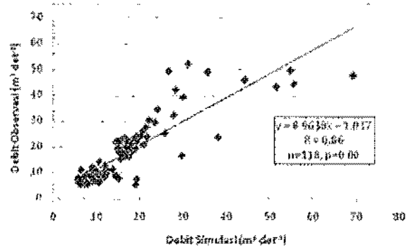
Gambar 4. Hidrograph aliran simulasi setelah proses validasi dan hidrograph observasi (bulan Februari-Maret tahun 2009 dan 2011)
