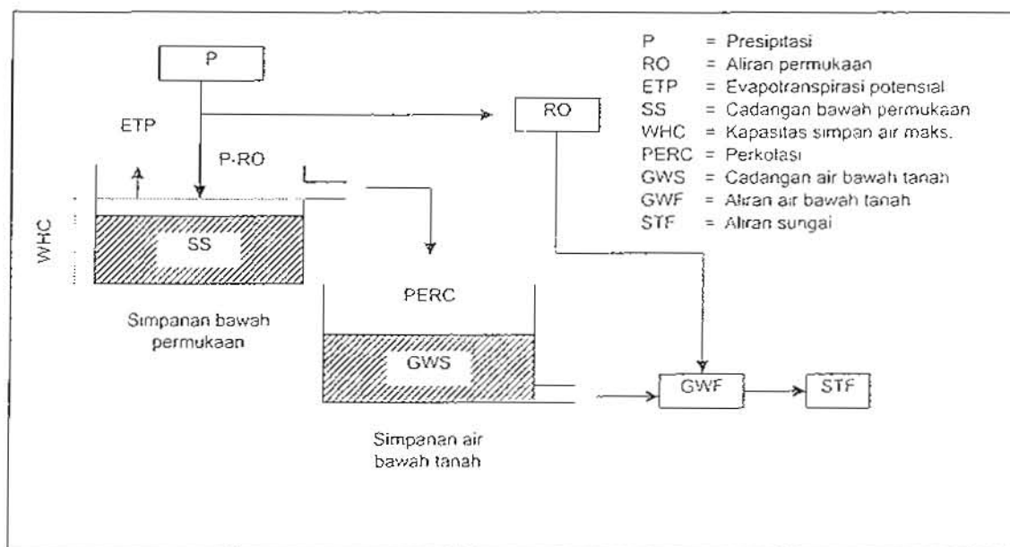
Gambar 1. Diagram alir MODDAS
