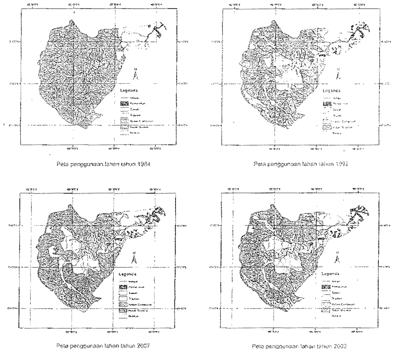
Gambar 4. Penggunaan lahan tahun 1984, 1992, 2002, dan 2007
