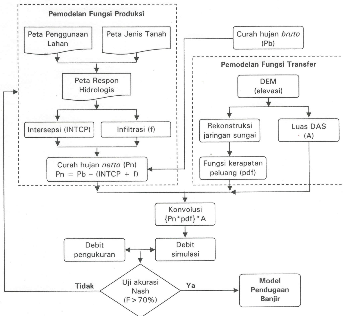
Gambar 2. Pemodelan fungsi produksi dan fungsi transfer
