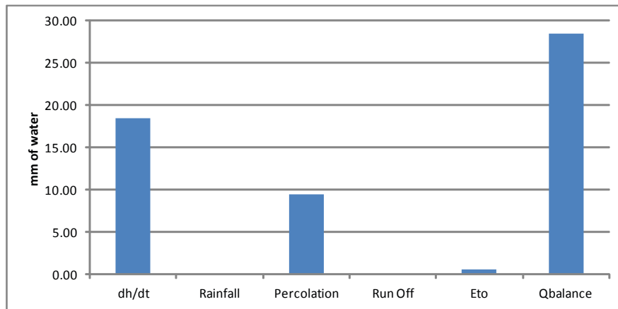
Gambar 9 Akumulasi komponen kesetimbangan air pada percobaan irigasi curah
