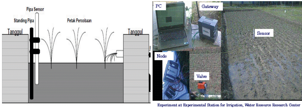
Gambar 4 Sistem irigasi genangan otomatis di lahan percobaan
