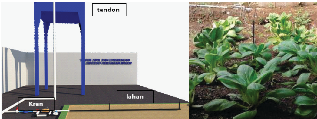
Gambar 5 Sistem irigasi curah otomatis di lahan percobaan
