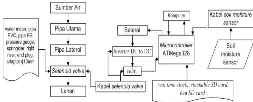
Gambar 2 Skema sistem irigasi curah otomatis
