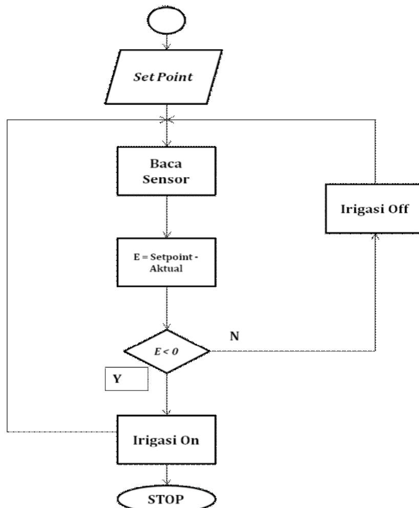
Gambar 3 Bagan alir algoritma pengendalian
