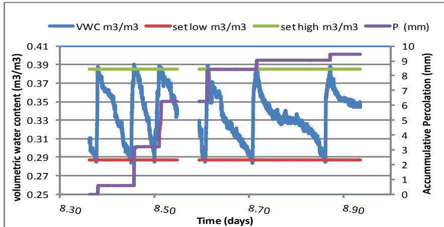
Gambar 8 Hasil percobaan irigasi otomatis untuk irigasi permukaan
