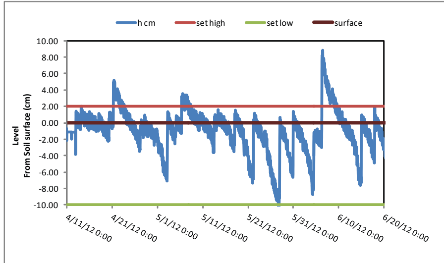
Gambar 6 Hasil percobaan irigasi otomatis untuk irigasi permukaan
