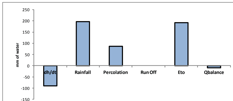
Gambar 7 Akumulasi komponen kesetimbangan air pada percobaan irigasi permukaan
