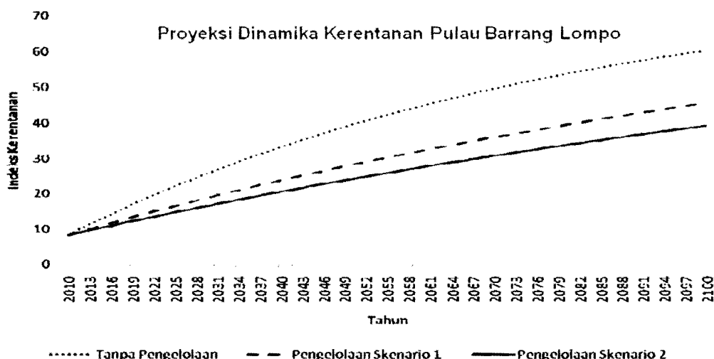
Gambar 1. Proyeksi kerentanan Pulau Barrang Lompo
