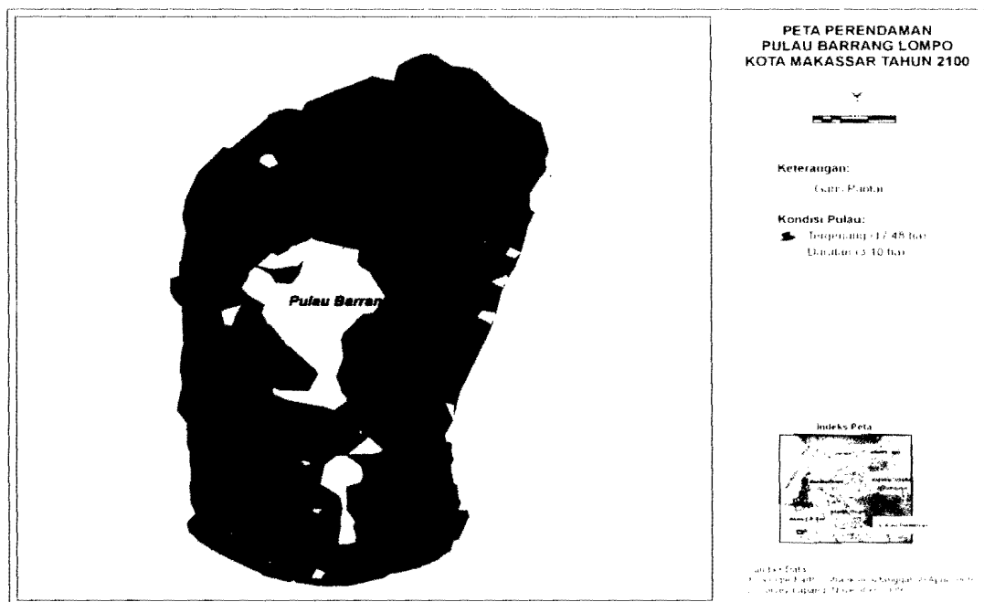
Gambar 2. Perkiraan kondisi daratan Pulau Barrang Lompo Tahun 2100
