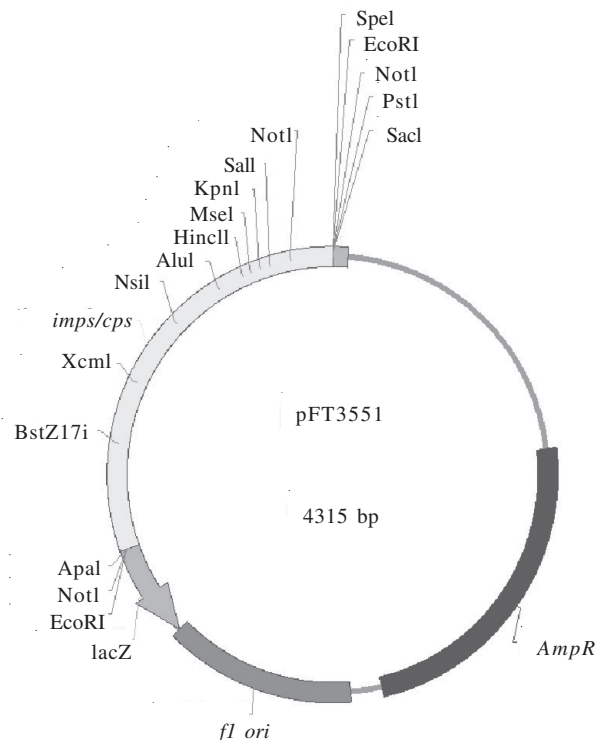
Fig 2 Plasmid pFT3551.
