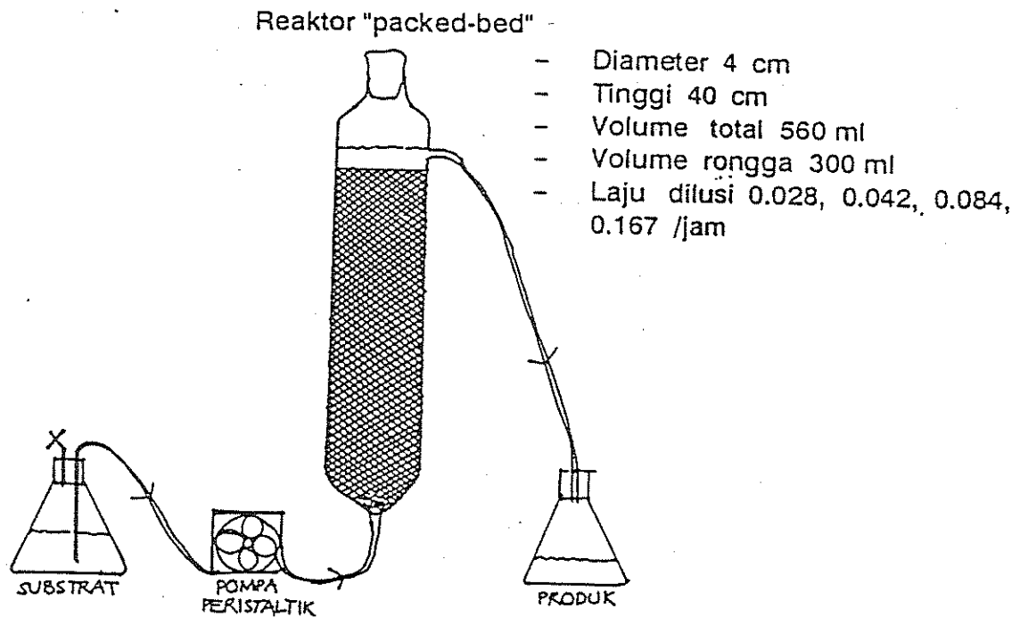
Gambar 2. Fermentasi sinambung.
