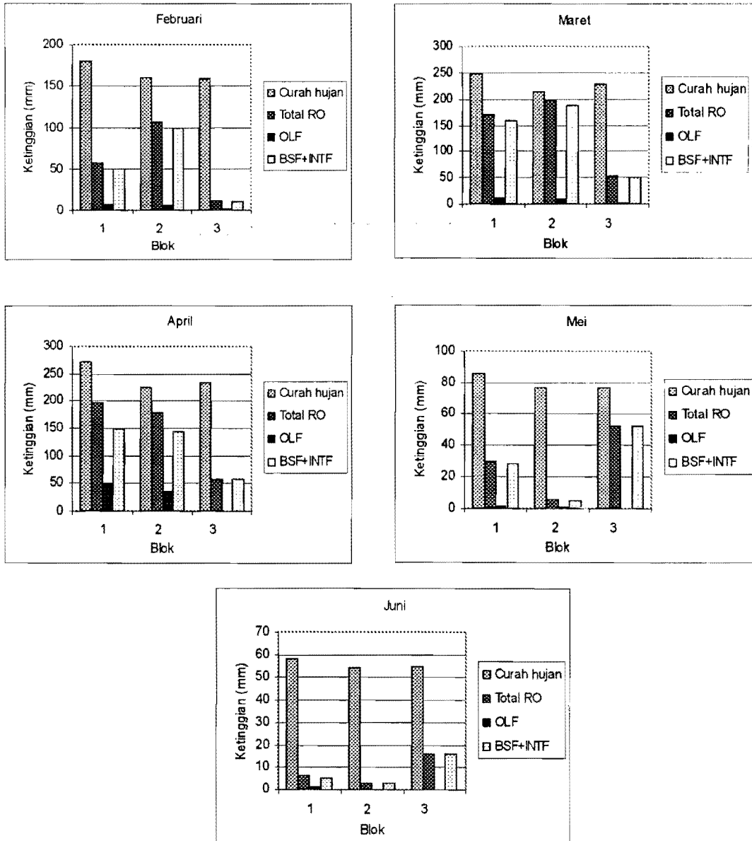
Gambar 2. Proporsi curah hujan yang menjadi komponen hidrograf
