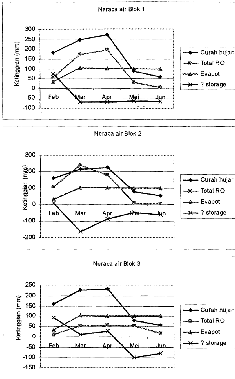
Gambar 3. Grafik neraca air pada setiap blok penelitian
