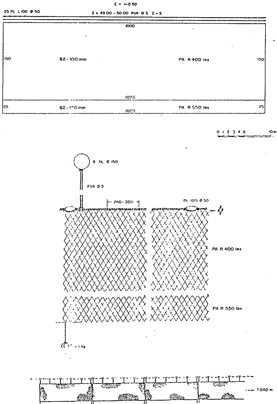
Gambar 15 Jaring insang hanyut untuk menangkap Spanish mackerel di Thailand (FAO, 1975).
