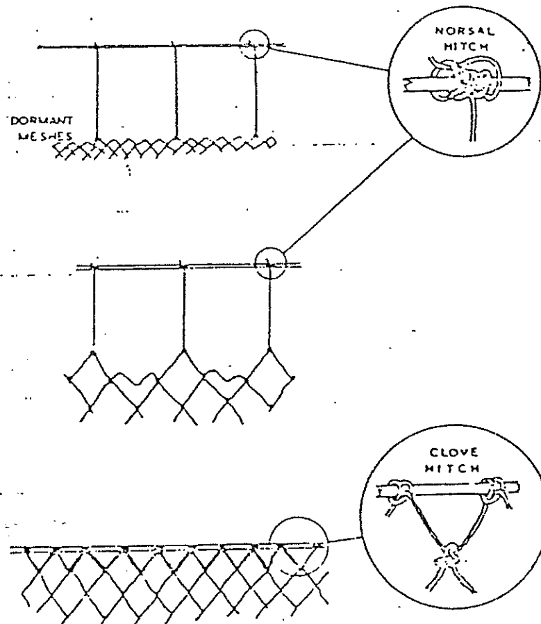
Gambar 8 Menggantungkan jaring pada ropes untuk jaring insang hanyut (GARNER, 1967)
