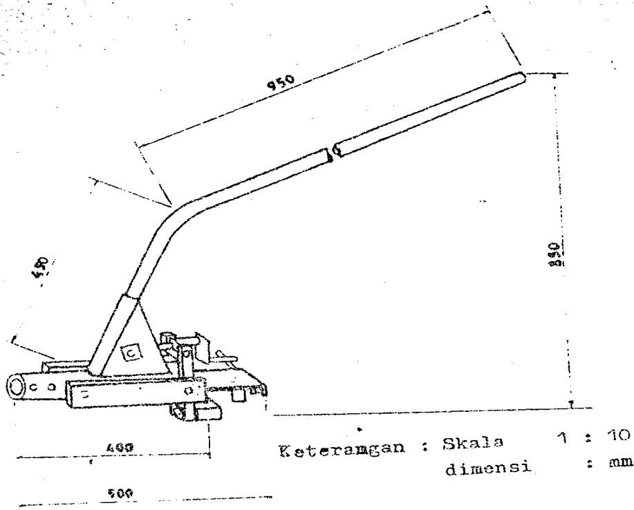
Gambar 1. Rangka "KANOL Y" yang asli
