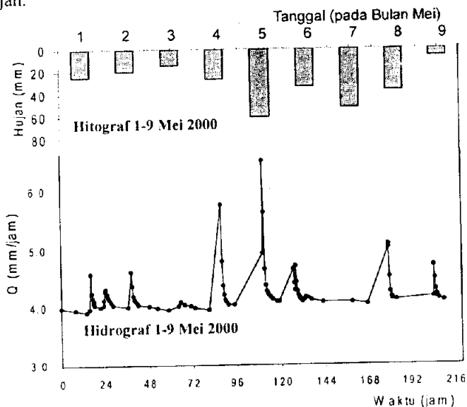
Gambar 2. Hietograf dan hydrograf aliran tanggal 1-9 Mei 2000
