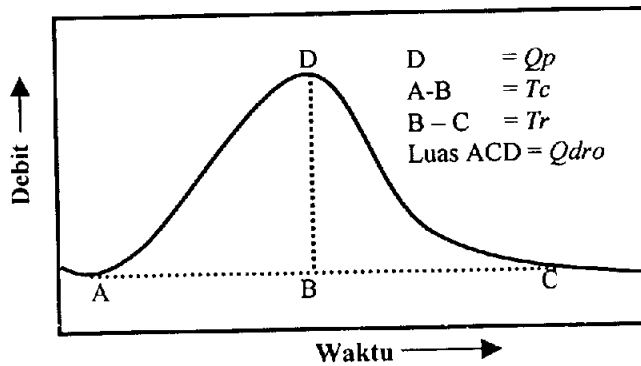
Gambar 1. Hidrograf aliran
