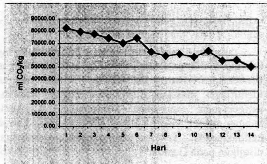
Gambar 2. Grafik pola respirasi bunga potong lili obductal pink
