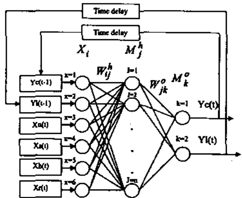
Gambar 1. Arsitektur JST respon dinamik
