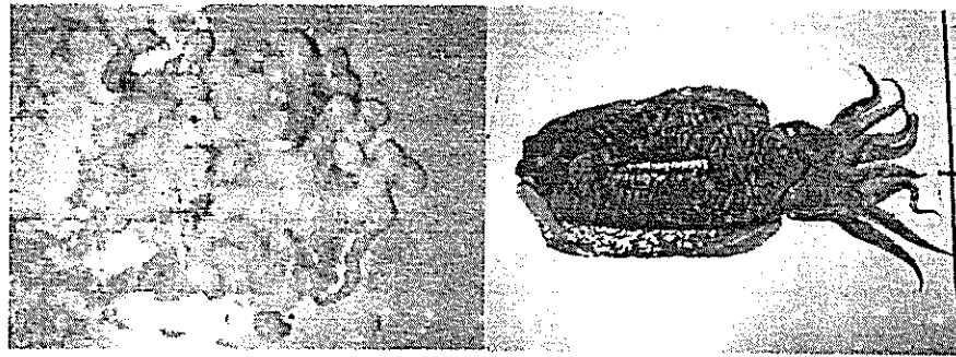
Gambar 5. Contoh telur cumi-cumi dan cumi-cumi dewasa yang di temukan di atraktor
