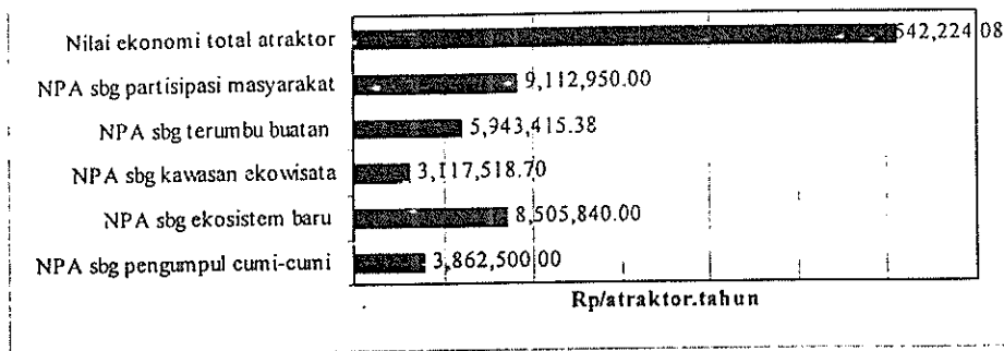
Gambar 6. Nilai potensi atraktor (NPA) cumi-cumi
