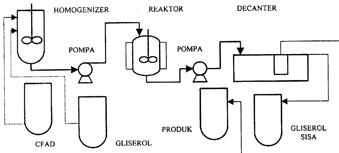
Gambar 1. Rancangan reaktor dan diagram alir
