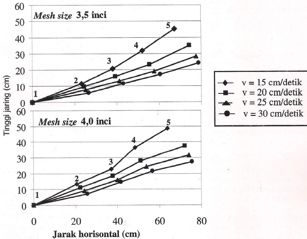
Gambar 6. Tinggi jaring goyang dengan ukuran mata 3,5 dan 4,0 inci pada berbagai kecepatan arus. Figure 6. Net height of jaring goyang with 3.5 and 4.0 inch mesh sizes at various current speed.
