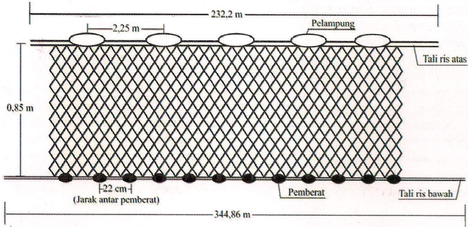
Gambar 2. Konstruksi jaring goyang yang digunakan oleh nelayan. Figure 2. Construction of jaring goyang used by fisherman.
