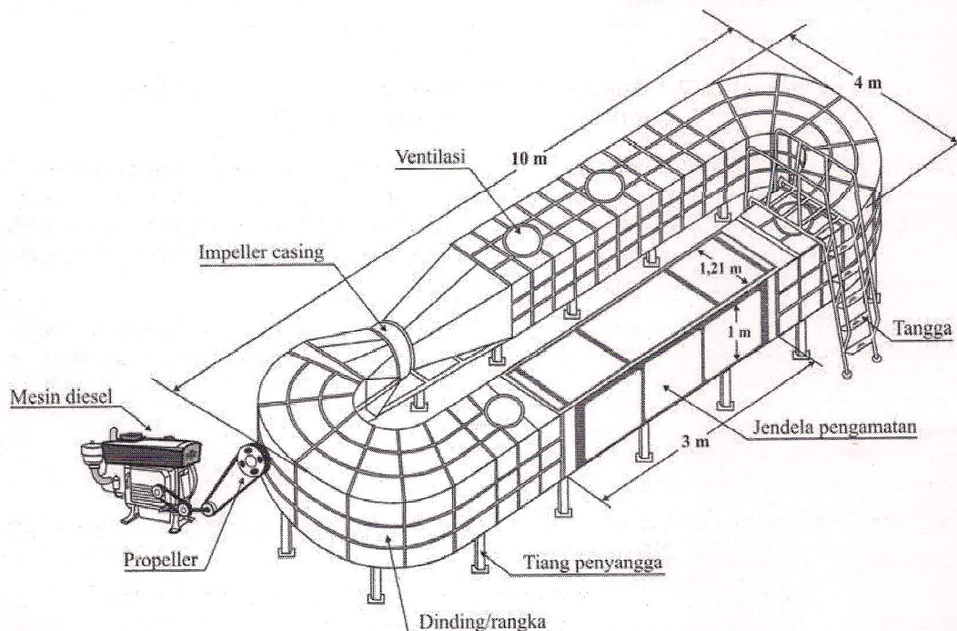
Gambar 1. Dimensi flume tank milik Departemen Pemanfaatan Sumber Daya Perikanan, Fakultas Perikanan dan Ilmu Kelautan, Institut Pertanian Bogor.
