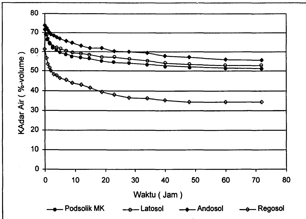
Gambar 2. Kadar air Tanah Menurut Waktu Setelah Tanah Jenuh Sempurna dan Dibiarkan bebas terdrainase
