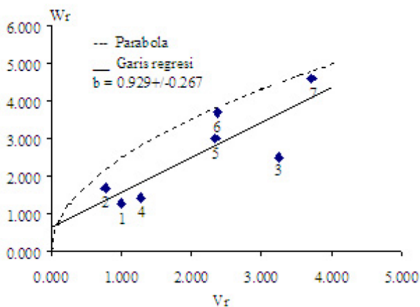
Gambar 1. Grafik regresi ragam peragam ( V_r , W_r ) dari analisis dialel 7 \times 7 untuk karakter jumlah anakan produktif. Seri silangan T. x T. 1. Situgintung, 2. Jatiluhur, 3. Gajah Mungkur, 4. B8503E-TB-9-0-3, 5. Krowal, 6. CT6510-24-1-3, 7. IR 64.
