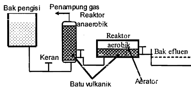
Gambar 1. Rancangan reaktor pengolahan limbah tekstil sistem kombinasi anaerobik-aerobik menggunakan biofilm konsorsium bakteri
