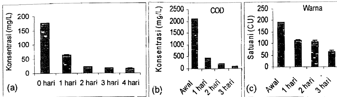
Gambar 4. Perombakan limbah tekstil buatan menggunakan biofilm konsorsium bakteri. (a) penurunan konsentrasi zat warna pada reaktor anaerobik sedangkan (b) dan (c) penurunan COD dan warna pada reaktor aerobik.
