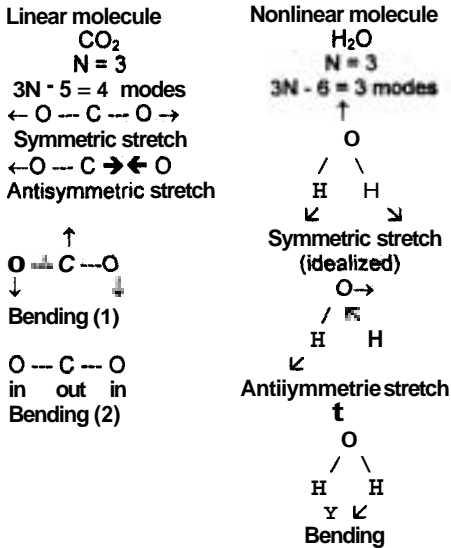
Gambar 1. Skema diagram vibrasi cara biasa untuk molekul linier CO_2 dan molekul linier (bent molecule) H_2O .
