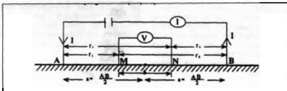
Gambar 3. Konfigurasi Elektroda Schlurnberger (Todd, D.K. 1995)
