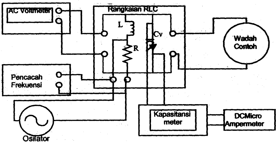
Gambar 2. Skema alat ukur nilai sifat dielektrik.
