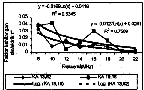
Gambar 15. Grafik pengaruh frekuensi terhadap rata-rata nilai faktor kehilangan dielektrik ( \epsilon'' ) pada kadar air 13,82 % dan 19,18 %
