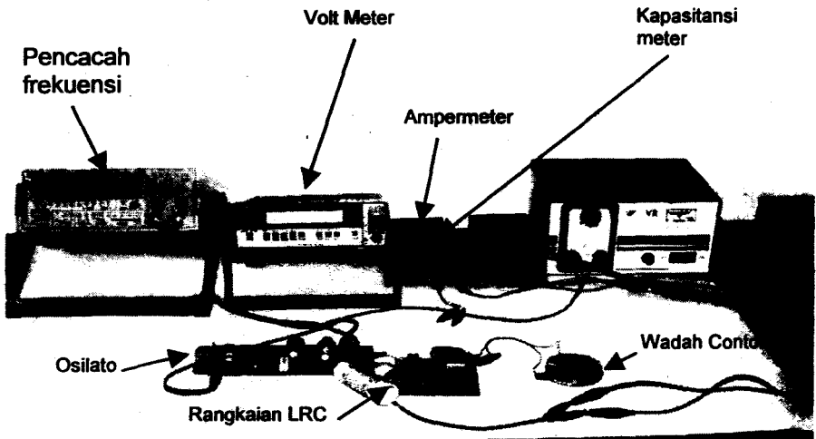
Gambar 4. Alat ukur nilai sifat dielektrik.
