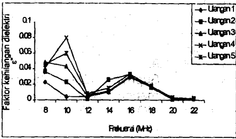
Gambar 13. Grafik pengaruh frekuensi terhadap nilai faktor kehilangan dielektrik ( \epsilon'' ) pada kadar air 19,18 %
