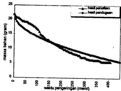
Gambar 4. Perbandingan massa bahan antara hasil pengukuran dengan hasil pendugaan
