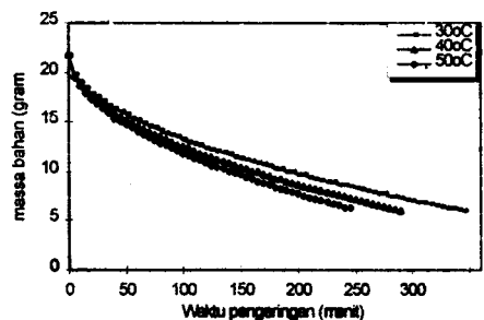
Gambar 8. Grafik penurunan massa bahan pada suhu sublimasi 30°C, 40°C dan 50°C
