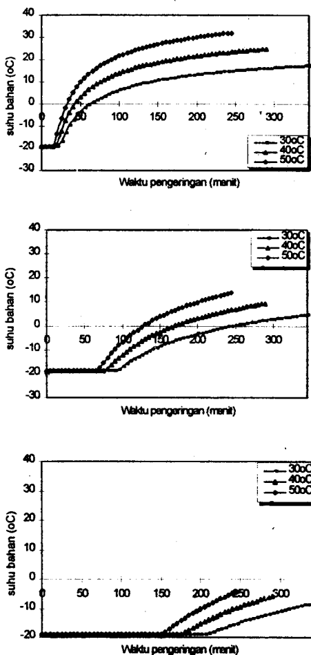
Gambar 6. Simulasi pergerakan suhu bahan (berturut-turut dari atas ke bawah: suhu bagian atas, tengah dan bawah) dengan suhu permukaan terkendali pada 30°C, 40°C dan 50°C.
