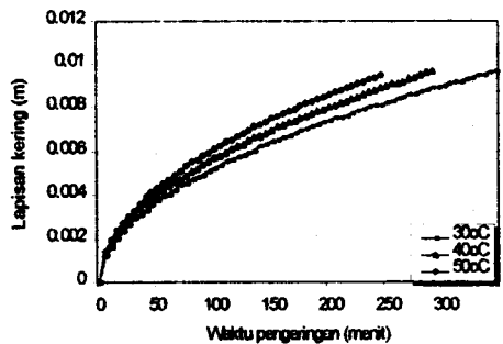
Gambar 10. Pergerakan lapisan kering bahan pada suhu sublimasi 30°C, 40°C dan 50°C
