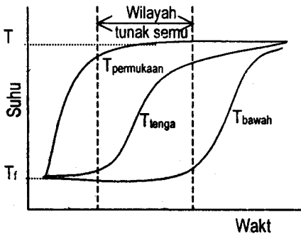
Gambar 7. Tipologi profil suhu pada proses pengeringan beku
