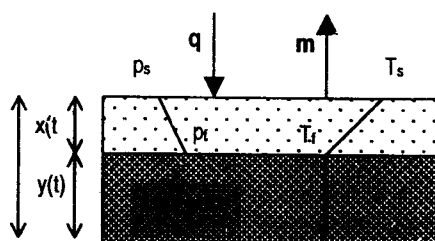
Gambar 2. Retreating Front Model pada proses pengeringan beku
