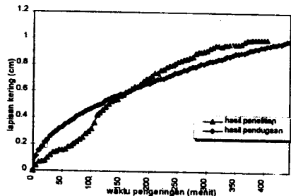
Gambar 5. Perbandingan pergerakan lapisan kering bahan antara hasil pengukuran dengan hasil pendugaan
