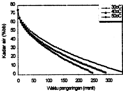
Gambar 9. Grafik penurunan kadar air bahan pada suhu sublimasi 30°C, 40°C dan 50°C
