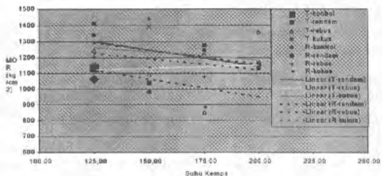
Gambar 3. Grafik Nilai Modulus of Elasticity (MOE) (1) dan Modulus of Rupture (MOR) (2) pada Kayu Agatis Solid dan Dipadatkan
