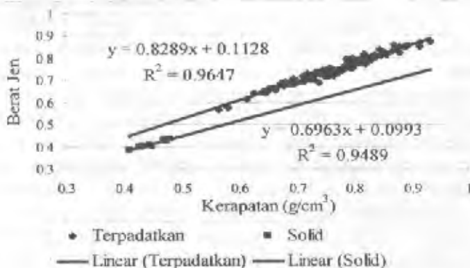
Gambar 2. Analisis Regresi Hubungan antara Kerapatan dan Berat Jenis pada Kayu Agatis Solid dan Terpadatkan
