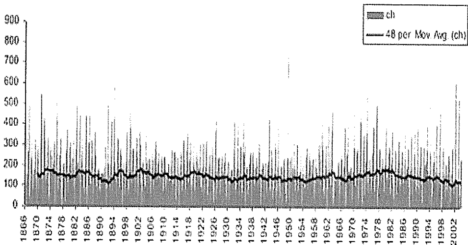
Gambar 4. Curah Hujan Bulanan Jakarta tahun 1866-2003 (sumber: WMO).
