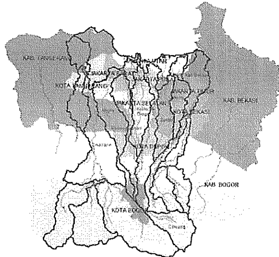
Gambar 7 Pembagian DAS di wilayah Jabodetabek
