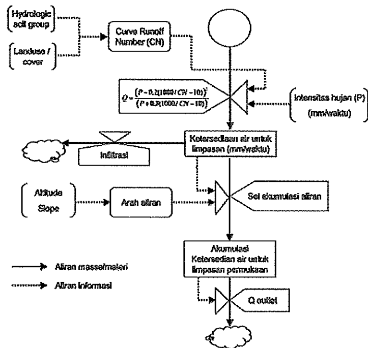
Gambar 2. skema penentuan run off di Jabodetabek
