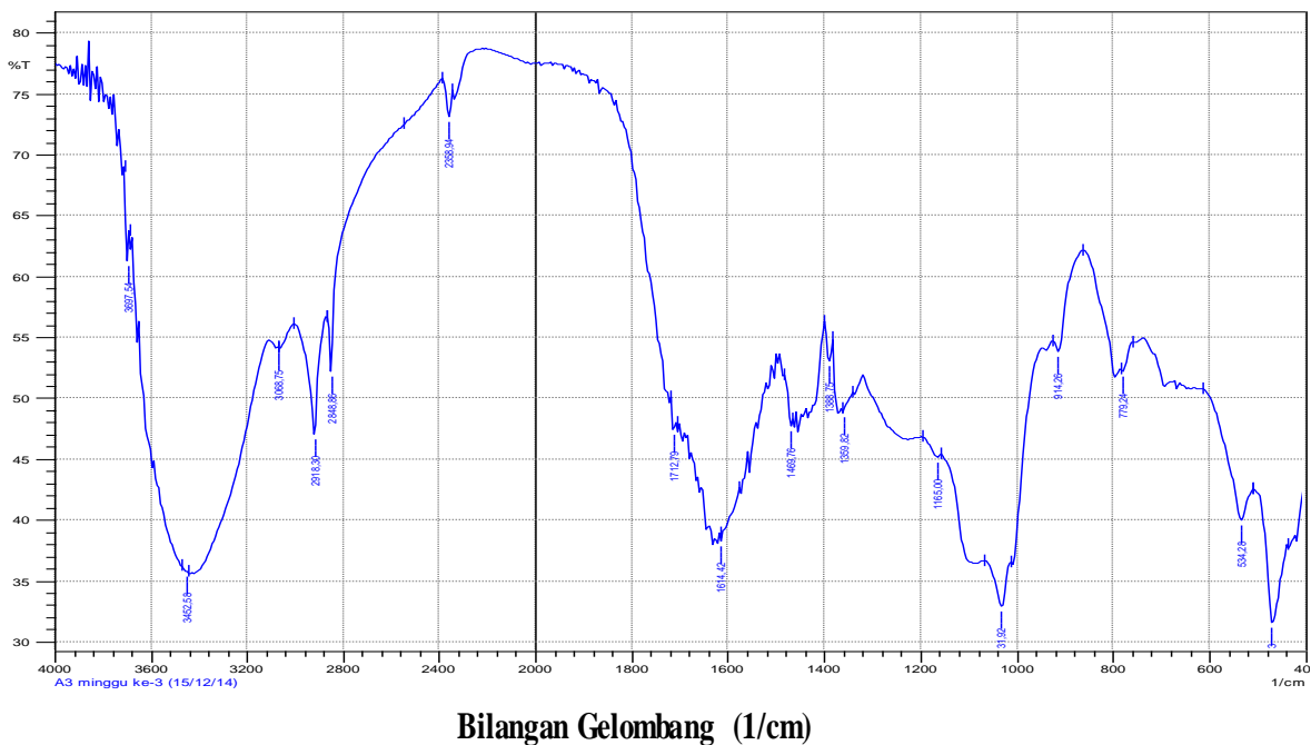
Gambar 6. Spektrum FTIR untuk perlakuan A3 hari ke-28 Figure 6. FTIR spectra for A3 treatment on day 28
