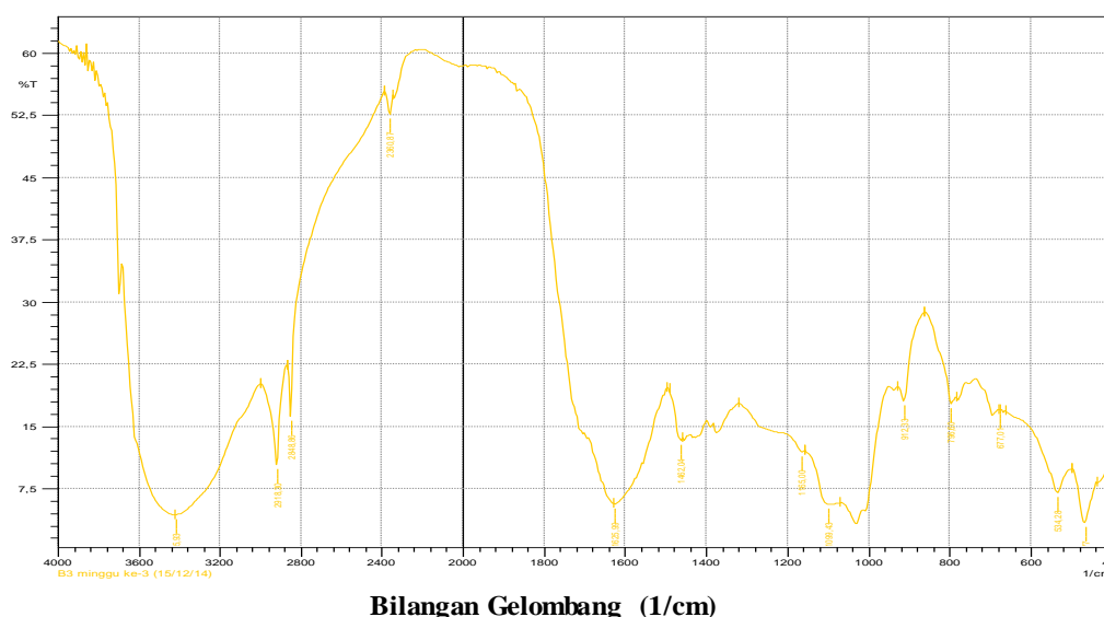
Gambar 7. Spektrum FTIR untuk perlakuan B3 hari ke-28
