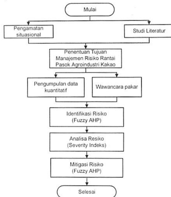
Gambar 1. Kerangka Fikir
