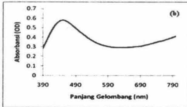
Gambar 4 (a) Pita transmitansi SiO 2 dan (b) absorbansi SiO 2 .
