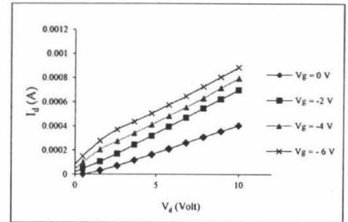
Gambar 6 Kurva I-V transistor film tipis.
