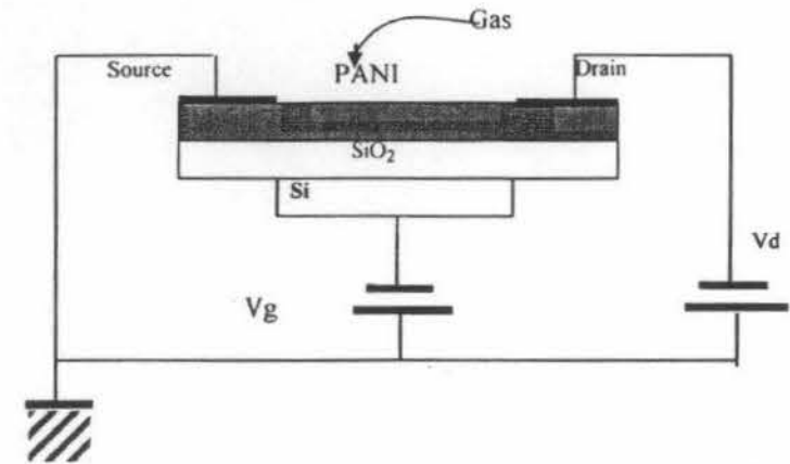
Gambar 2 Konfigurasi rangkaian listrik untuk sensor berbasis transistor film tipis
