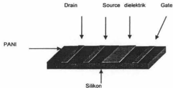
Gambar 1 Konfigurasi sensor berbasis transistor film tipis.
