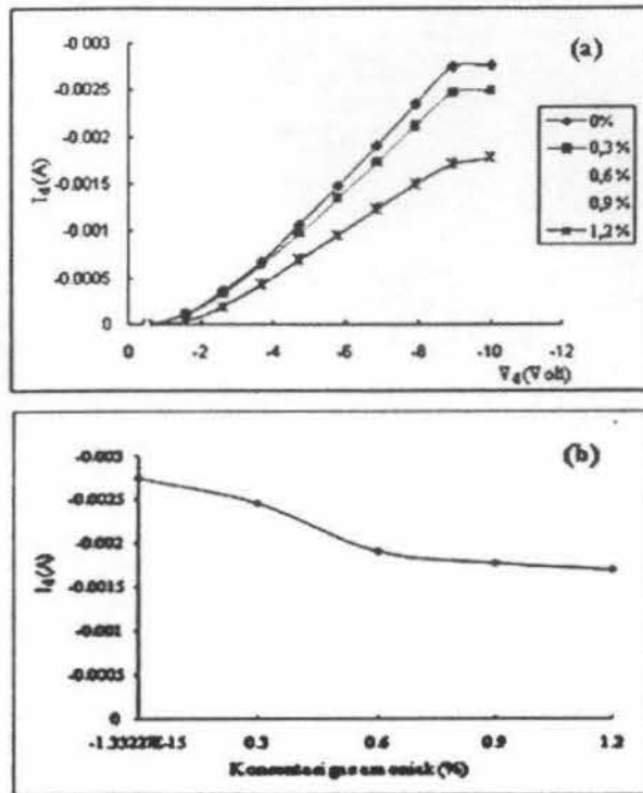
Gambar 7 (a) Pengaruh konsentrasi amoniak terhadap transistor film tipis organik, (b) pengaruh konsentrasi gas amoniak terhadap arus drain ( V_d = 8,9 Volt)
