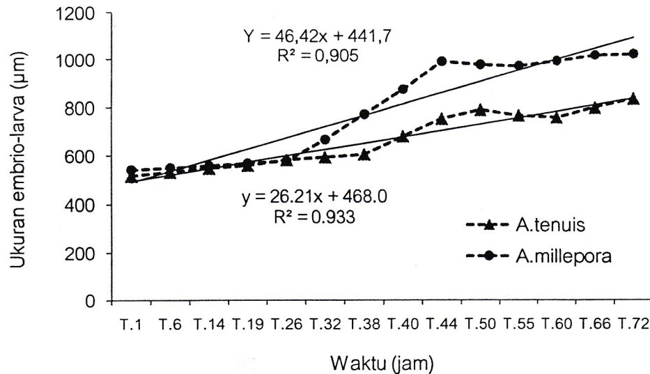
Gambar 1. Perkembangan ukuran embrio dan larva Acroporidae ( A. tenuis dan A. millepora ).
