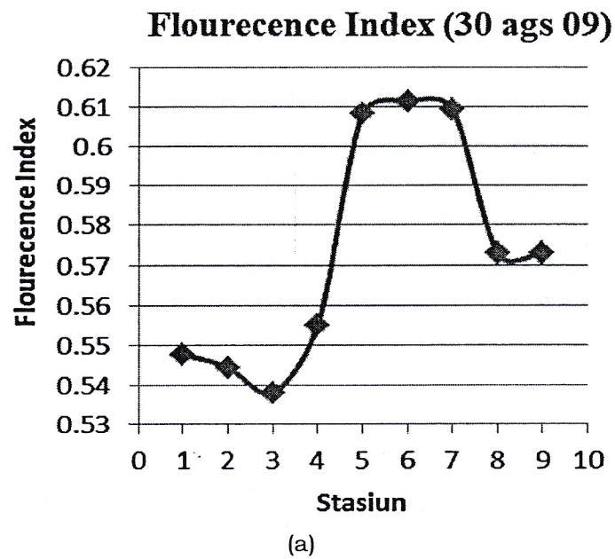
Gambar 6. (a). Hasil pemrosesan dengan Algoritma Fluorescence Index 30 Agustus 2009
