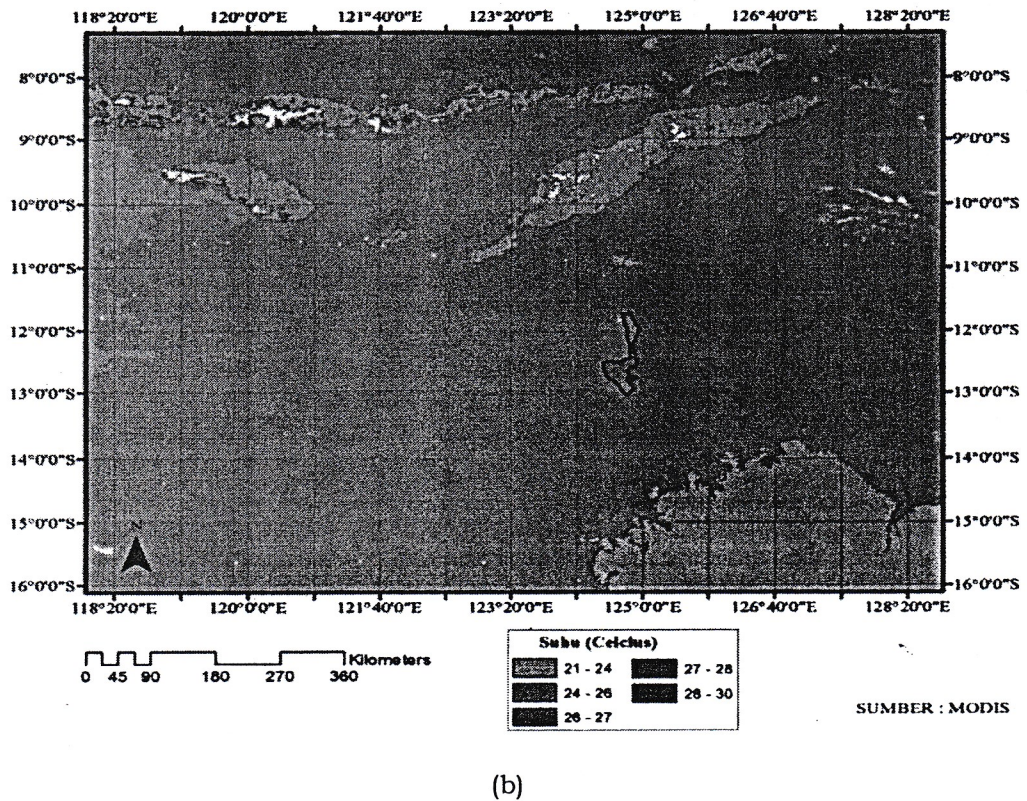
Gambar 7. SST hasil algoritma Callison dari citra MODIS, (a) 30 Agustus 2009, (b) 8 September 2009
