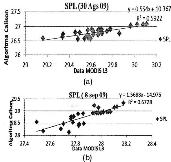
Gambar 8. Korelasi linear yang dihasilkan antara algoritma SST Calison dengan data citra MODIS level 3, (a) 30 Agustus 2009, (b) 8 September 2009
