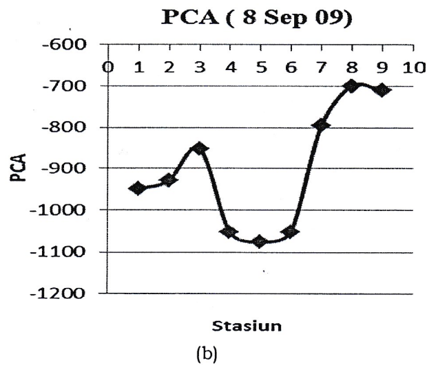
Gambar 3. (b). Hasil pemrosesan dengan algoritma PCA 8 September 2009
