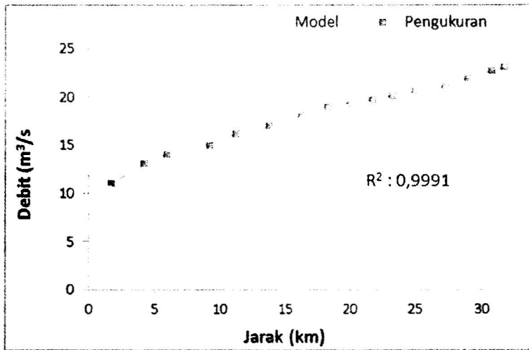
Gambar 5 Perbandingan debit model dengan hasil pengukuran di lapangan
