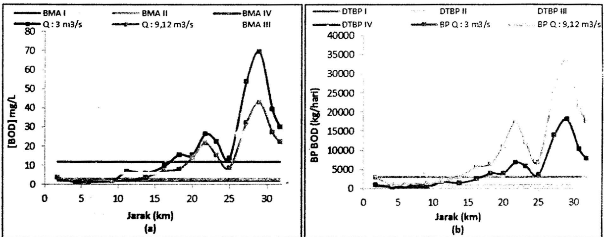
Gambar 10 Hasil simulasi skenario 3 untuk nilai BOD (a) dan beban pencemaran (b).
