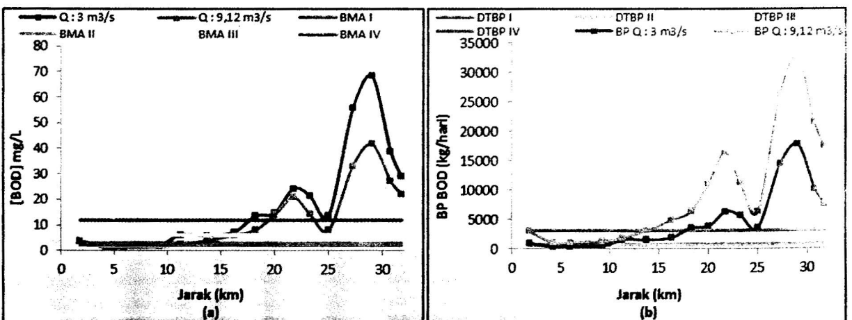
Gambar 11 Hasil simulasi skenario 4 untuk nilai BOD (a) dan beban pencemaran (b).
