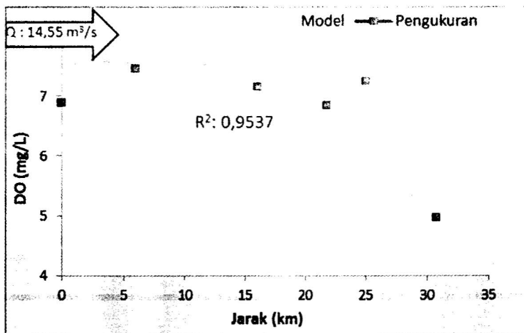
Gambar 6 Perbandingan nilai DO model dengan hasil pengukuran di lapangan
