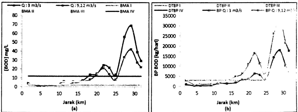
Gambar 8 Hasil simulasi skenario 1 untuk nilai BOD (a) dan beban pencemaran (b)
