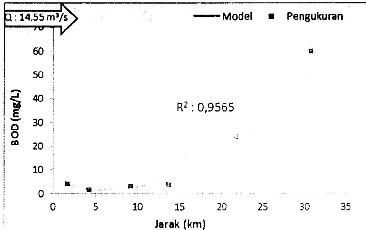
Gambar 7 Perbandingan nilai BOD model dengan hasil pengukuran di lapangan
