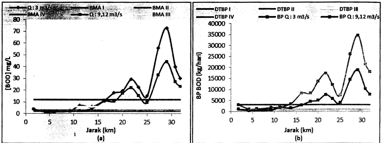
Gambar 9 Hasil simulasi skenario 2 untuk nilai BOD (a) dan beban pencemaran (b)
