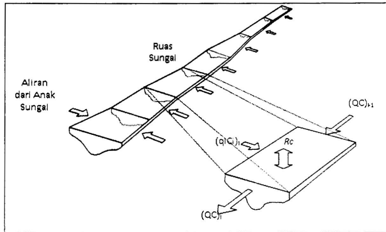
Gambar 1 Sistem pemodelan kualitas air finite segment
