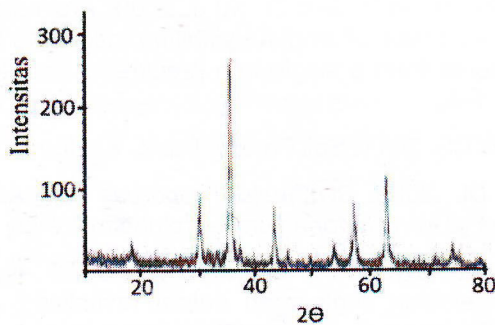
Gambar 1 Pola difraksi sinar-X nano-magnetit hasil sintesis.
