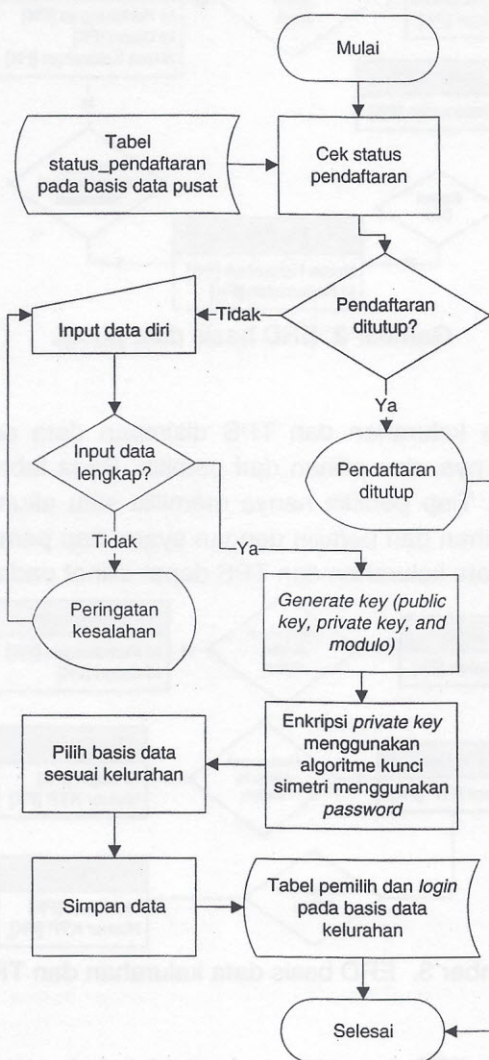
Gambar 4. Flowchart pendaftaran pemilih.
