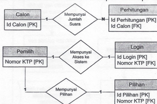
Gambar 3. ERD basis data kelurahan dan TPS.
