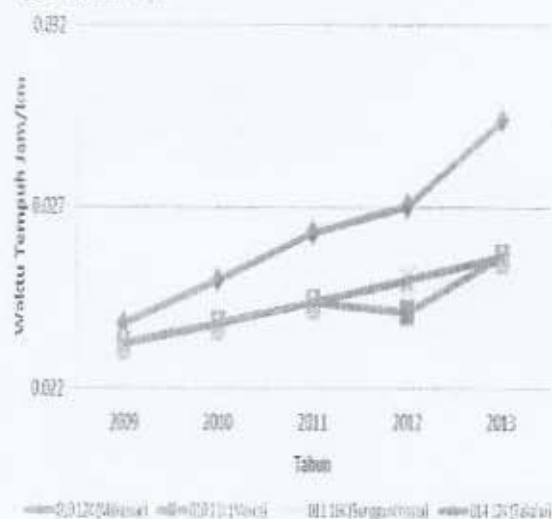
Gambar 8. Waktu tempuh ( Travel Time )
