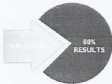
Gambar 3. Hukum Pareto
