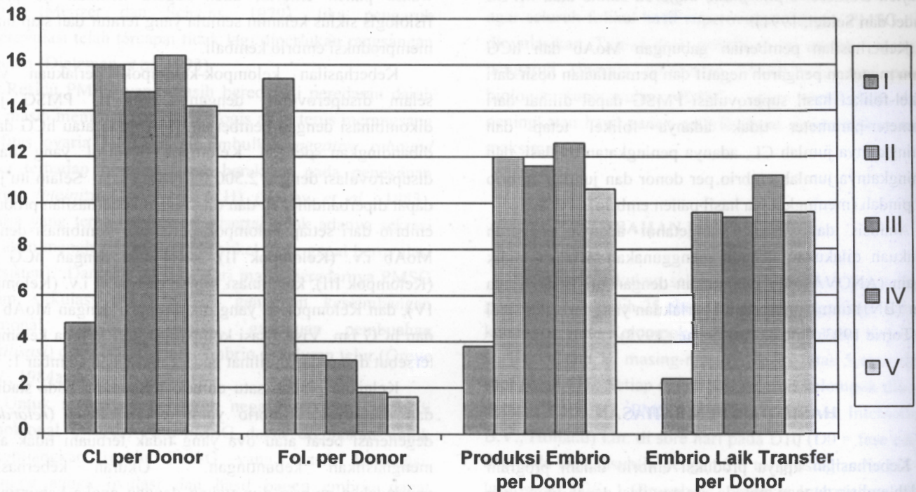
Gambar 1. Histogram Perbandingan Keberhasilan Kelima Kelompok Donor Yang Disuperovulasi 2.500 IU PMSG Dengan Atau Tanpa Kombinasi Perlakuan MoAb-hCG
