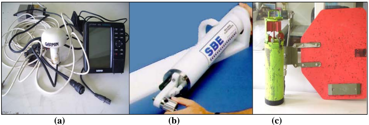
Gambar 2. Peralatan yang digunakan dalam survei lapang (a) GPS Garmin, (b) Tide Gauge SBE Type, dan (c) Aandera Current Meter tipe RCM 7
