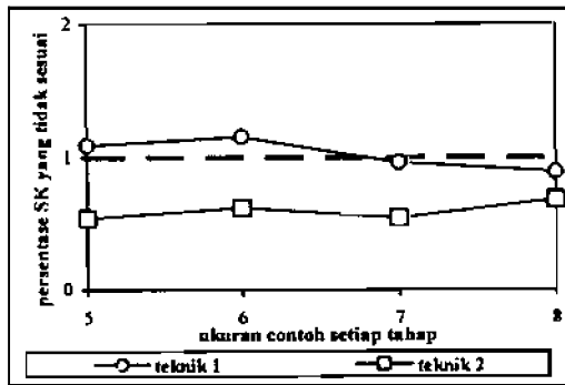
Gambar 3. Persentase selang kepercayaan 99% bagi nilai tengah yang tidak memuat \mu
