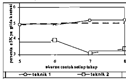
Gambar 2. Persentase selang kepercayaan 95% bagi nilai tengah yang tidak memuat \mu
