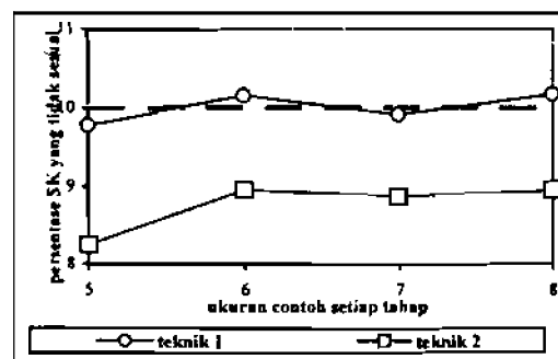
Gambar 1. Persentase selang kepercayaan 90% bagi nilai tengah yang tidak memuat \mu
