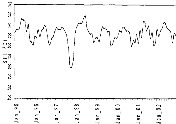
Gambar 2 Fluktuasi suhu permukaan laut di perairan Pulau Nias
