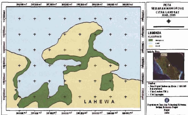
Gambar 9 Luasan hutan mangrove di Lahewa tahun 2005
