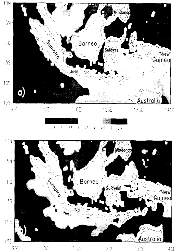
Gambar 3 Puncak ke puncak amplitudo SPL (a) variabilitas tahunan (b) variabilitas antartahun di Perairan Indonesia (Qu et al. 2005).
