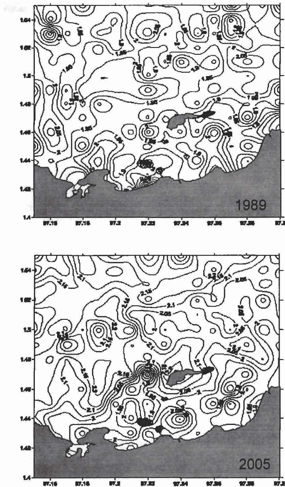
Gambar 6 Distribusi konsentrasi klorofil-a di sekitar pantai Lahewa tahun 1989 (atas) dan tahun 2005 (bawah)
