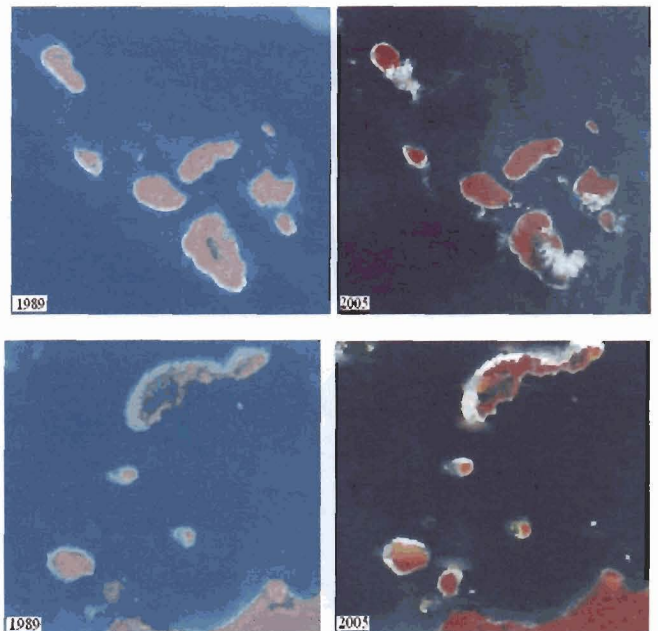
Gambar 11 Citra komposit 421 Landsat tahun 1989 dan 2005 di sebagian pulau-pulau kecil perairan Pulau Nias
