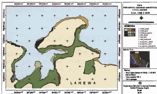
Gambar 10 Perubahan tutupan hutan mangrove antara tahun 1989 dan 2005 di Lahewa
