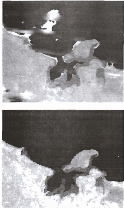
Gambar 7 Luasan tutupan mangrove di Lahewa (atas) dan Tuhemberu (bawah) pada tahun 1989 dan 2005
