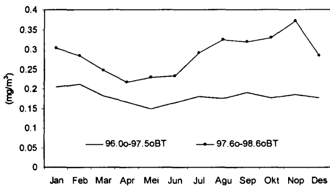
Gambar 5 Fluktuasi konsentrasi klorofil-a rata-rata bulanan di pantai barat dan timur (atas) dan rata-rata bulanan selama tahun 1997-2006 (bawah)
