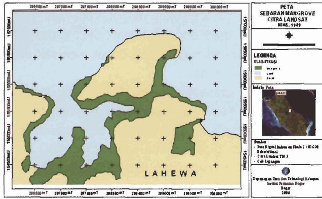
Gambar 8 Luasan hutan mangrove di Lahewa tahun 1989
