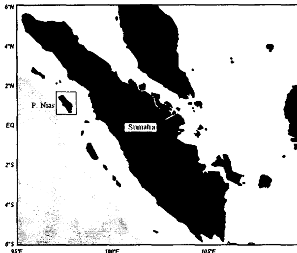
Gambar 1 Lokasi penelitian di perairan Pulau Nias
