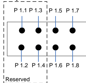
Gambar 6 Skema pin masukan.
