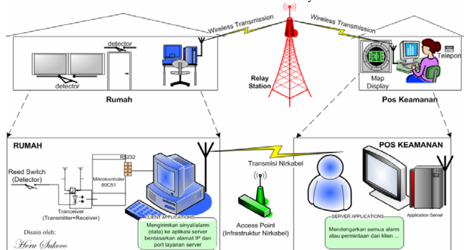
Gambar 1 Arsitektur sistem keamanan perumahan SIJELITA lama.
