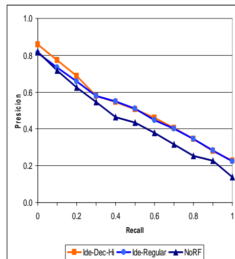
Gambar 2 Kurva recall-precision RG10 dan DH10 pada iterasi ke-1.
