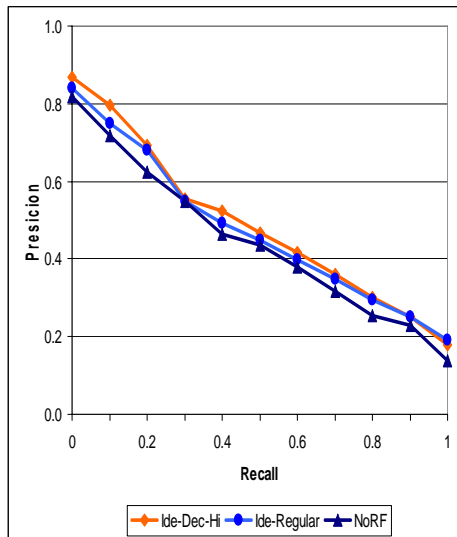
Gambar 3 Kurva recall-precision RG5 dan DH5 pada iterasi ke-2.
