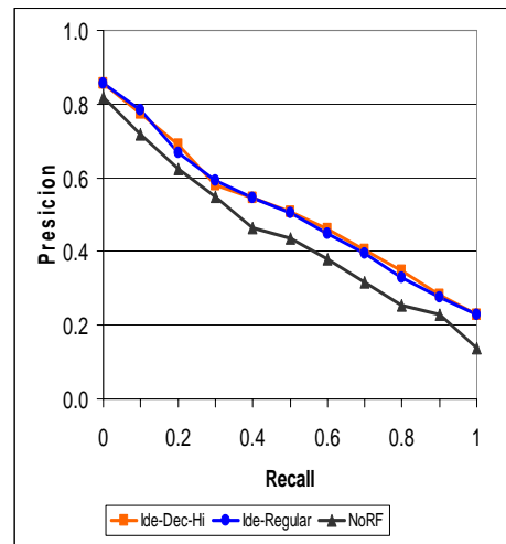
Gambar 1 Kurva recall-precision RG5 dan DH5 pada iterasi ke-1.
