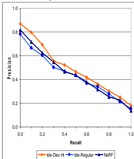
Gambar 4 Kurva recall-precision RG10 dan DH10 pada iterasi ke-2.
