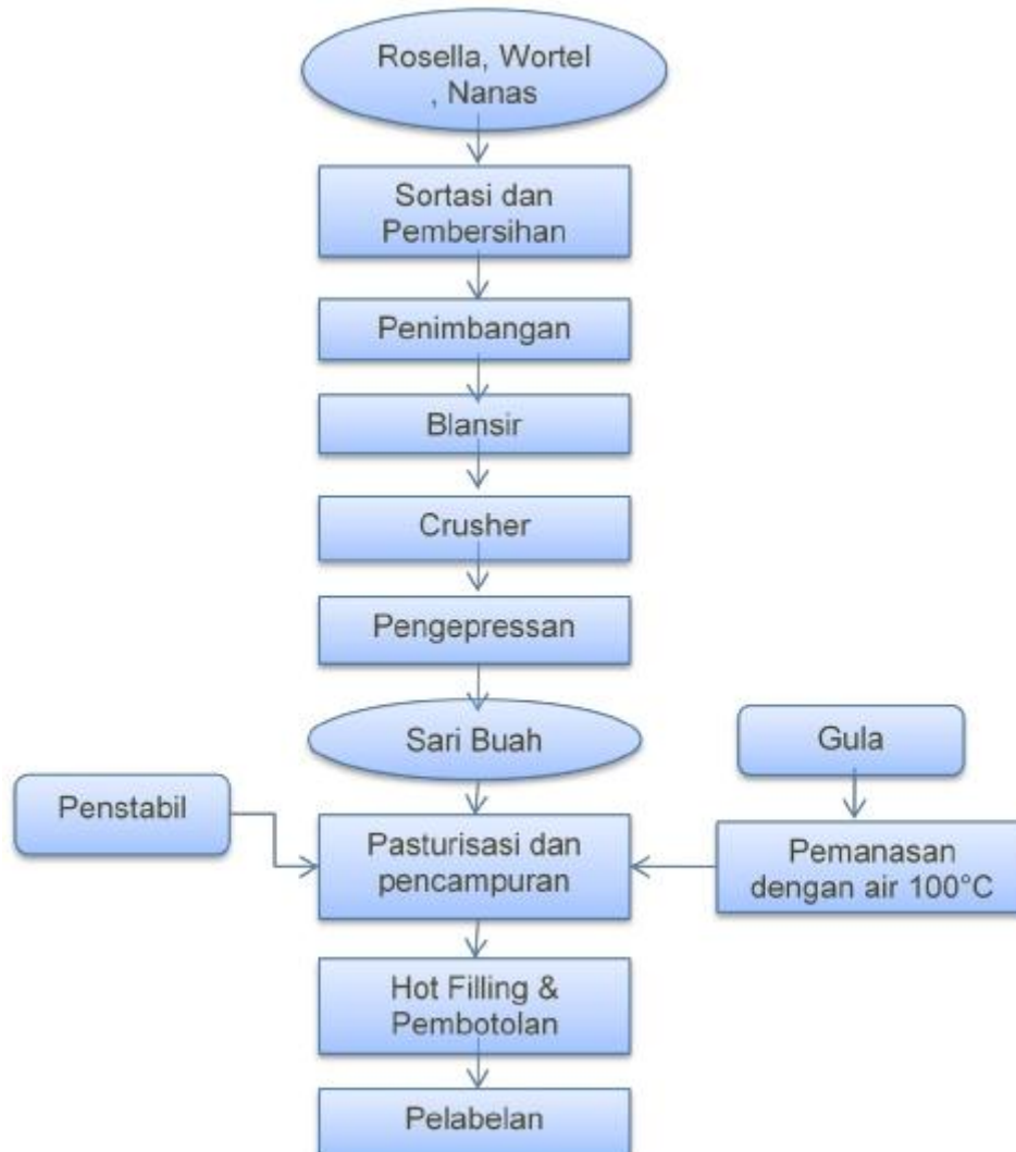
Gambar 1 Bagan alir produksi D'Bloem
