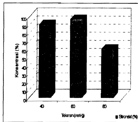
Gambar 7. Histogram kemurnian sitronelal dan waktu total proses hasil distilasi fraksionasi berbagai rasio refluks minyak sereh wangi.
