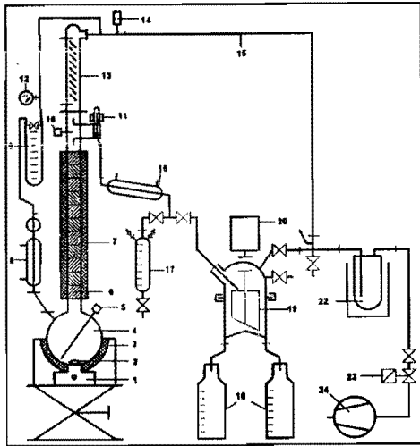
Gambar 2. Unit Alat Distilasi Fraksionasi Skala Bench
