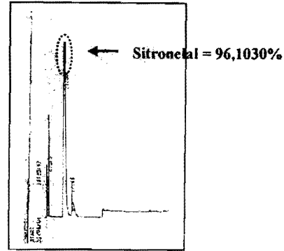
Gambar 6. Kromatogram Hasil Distilasi Fraksionasi Run 2 pada Fraksi 2
