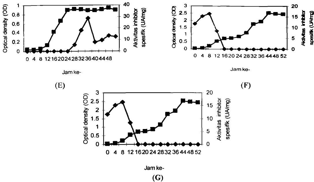
Gambar 5. Aktivitas inhibitor protease (UA/mg) dan optical density (OD), pH awal media 7 ( yeast extract 1% (A), 0,5% (B), 0,1% (C)); pH awal 8 ( yeast extract 1% (D), 0,5% (E), 0,1% (F)); dan MB+glukosa 0,05%; -■- OD dan -◆- aktivitas inhibitor protease (UA/mg)
