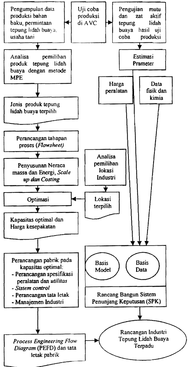
Gambar 1. Diagram Alir Penelitian Rancang Bangun Industri Tepung Lidah Buaya Terpadu
