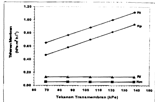
Gambar 5. Perubahan nilai komponen tahanan membran menurut fungsi tekanan transmbran pada laju alir umpan 2,97 m s^{-1}
