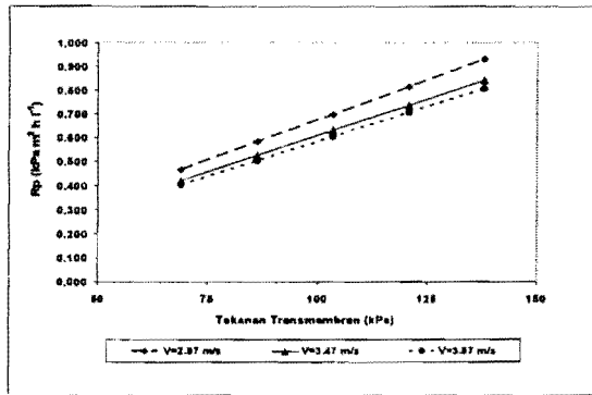
Gambar 4. Pengaruh tekanan transmbran terhadap tahanan polarisasi konsentrasi ( R_p )
