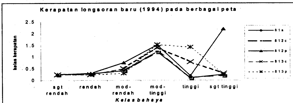
Gambar 5. Perbandingan hasil pemetaan tahun 1981 dengan cara berbeda yang diuji berdasarkan data longsorان tahun 1994
