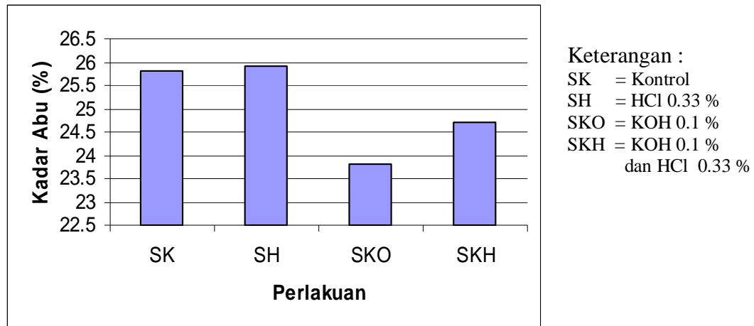
Gambar 3. Kadar abu Natrium alginat dari beberapa perlakuan perendaman rumput laut.
