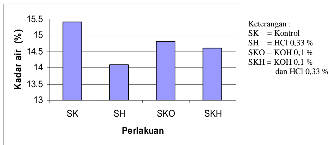
Gambar 2. Kadar air Natrium alginat dari beberapa perlakuan perendaman rumput laut.
