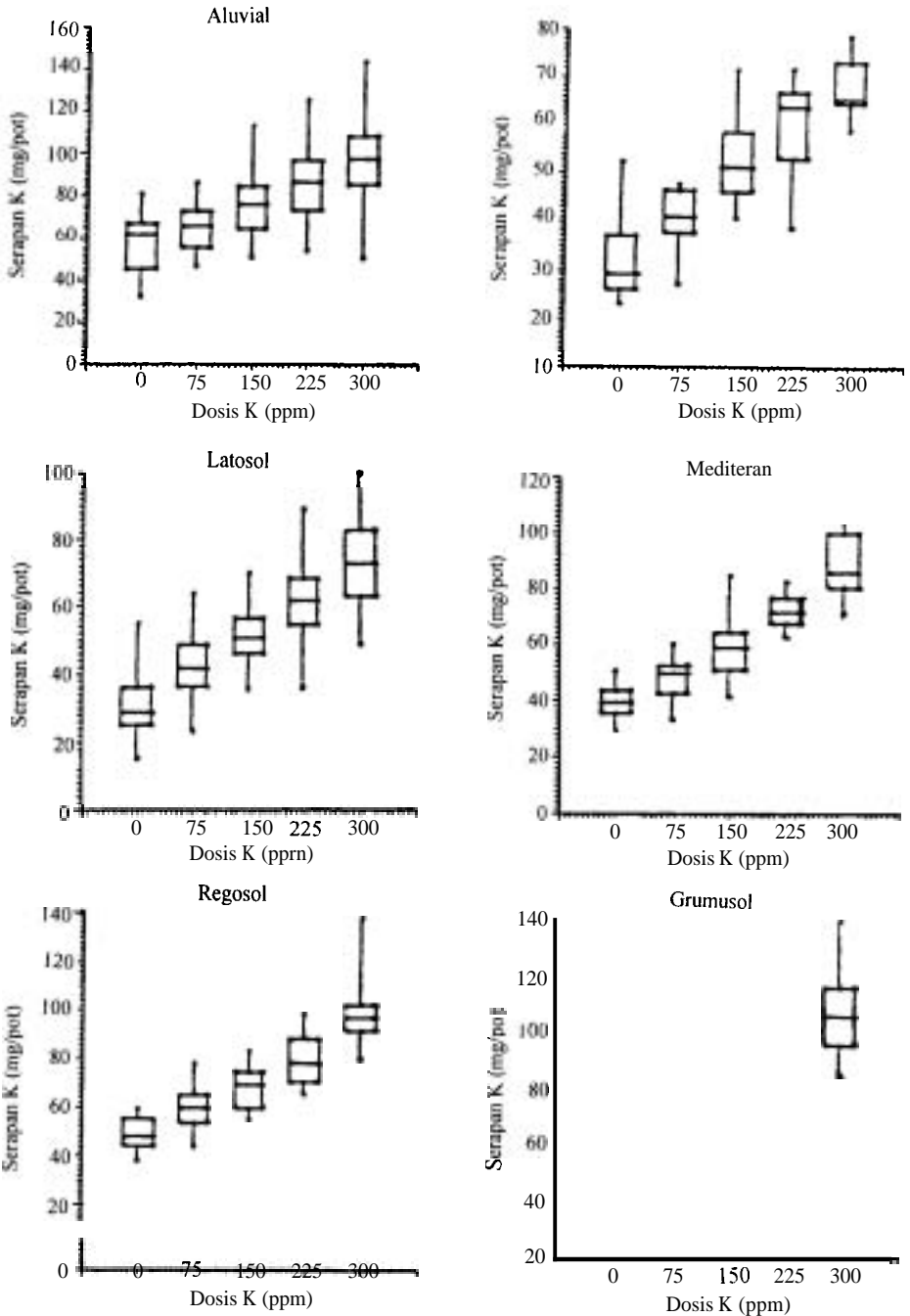
Gambar 3. Plot Kuantil untuk Sabuk 95% dan Garis Median untuk Regresi Grup Data dengan K-tanah sebagai Peubah Konkomitan
